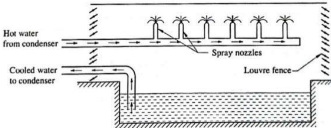
Fig : Spray ponds
